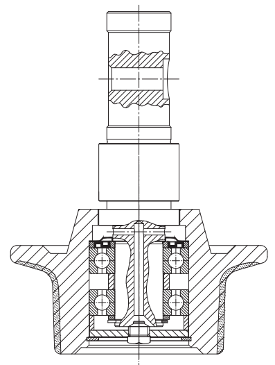
Aufbau Laufrolle mit Steckachse
