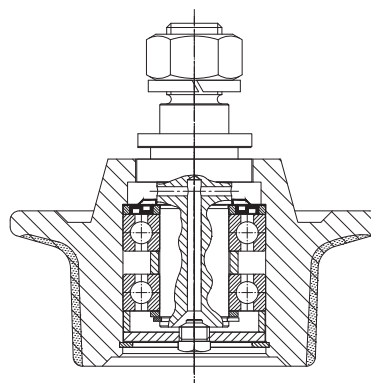
Aufbau Laufrolle mit Gewindeachse
