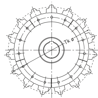
HEKO Kettenrad GTA
