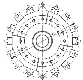
HEKO Kettenrad GIA
